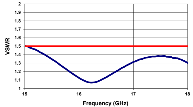
VSWR ( 15-18 GHz )
