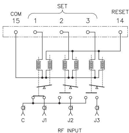
RF INPUT
