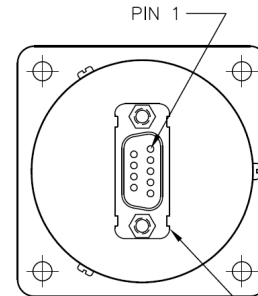
D-Sub 9-PIN D-SUB MINI CONNECTOR
