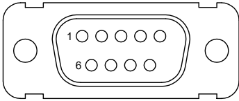
“-S OPTION” 9-PIN D-SUB CONNECTOR (Example: CCR-33K10-S)
