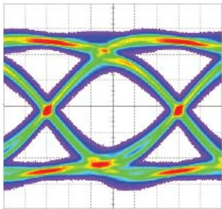
GRF121 @ 28Gbps
