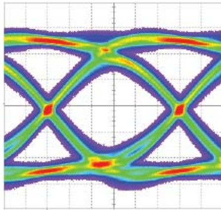
GRF121 @ 28Gbps
